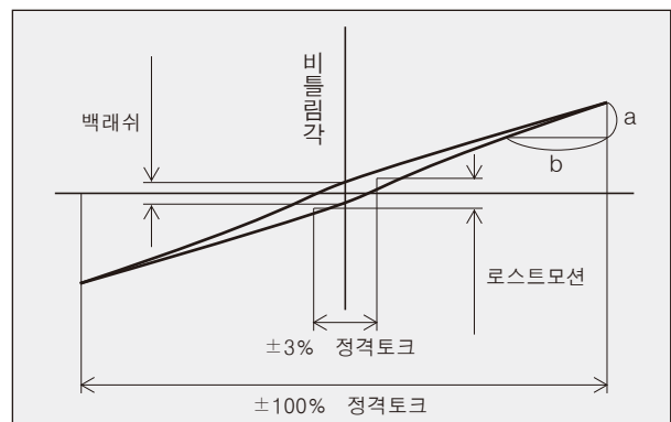
〈히스테리시스 곡선〉
